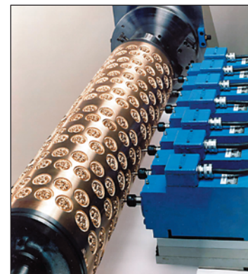
APV Baker Die
